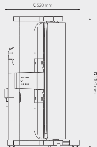
Vorderansicht, zusammengeklappt
